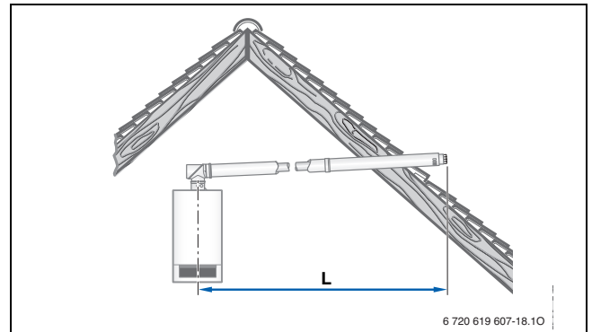
Res. 18 WH/WS baca kiti ile montaj varyasyonları (C 13x )
