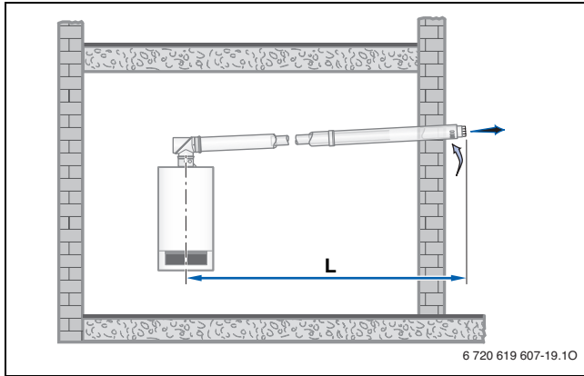
Res. 16 WH/WS baca kiti ile montaj varyasyonları (C 13x )
