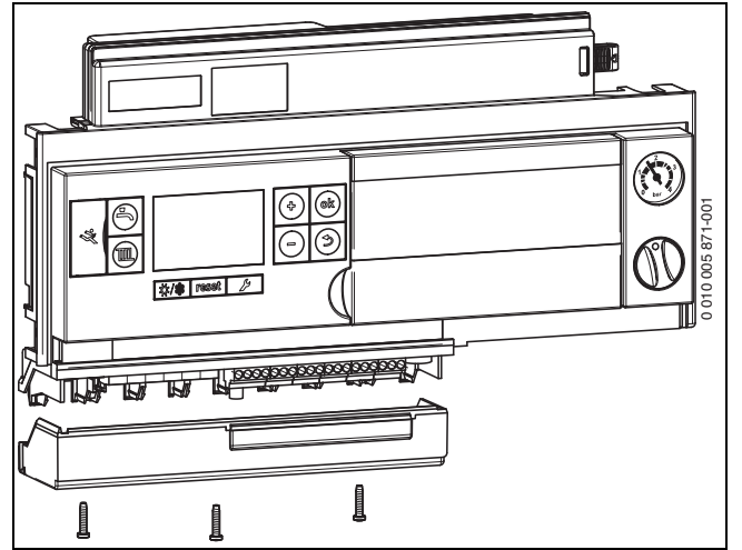
Res. 25 Kapağın sökülmesi
