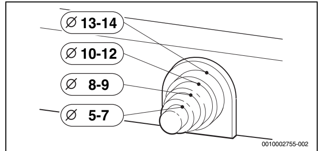
Res. 26 Sabitleme bandının kablo çapına uygun ayarlanması
