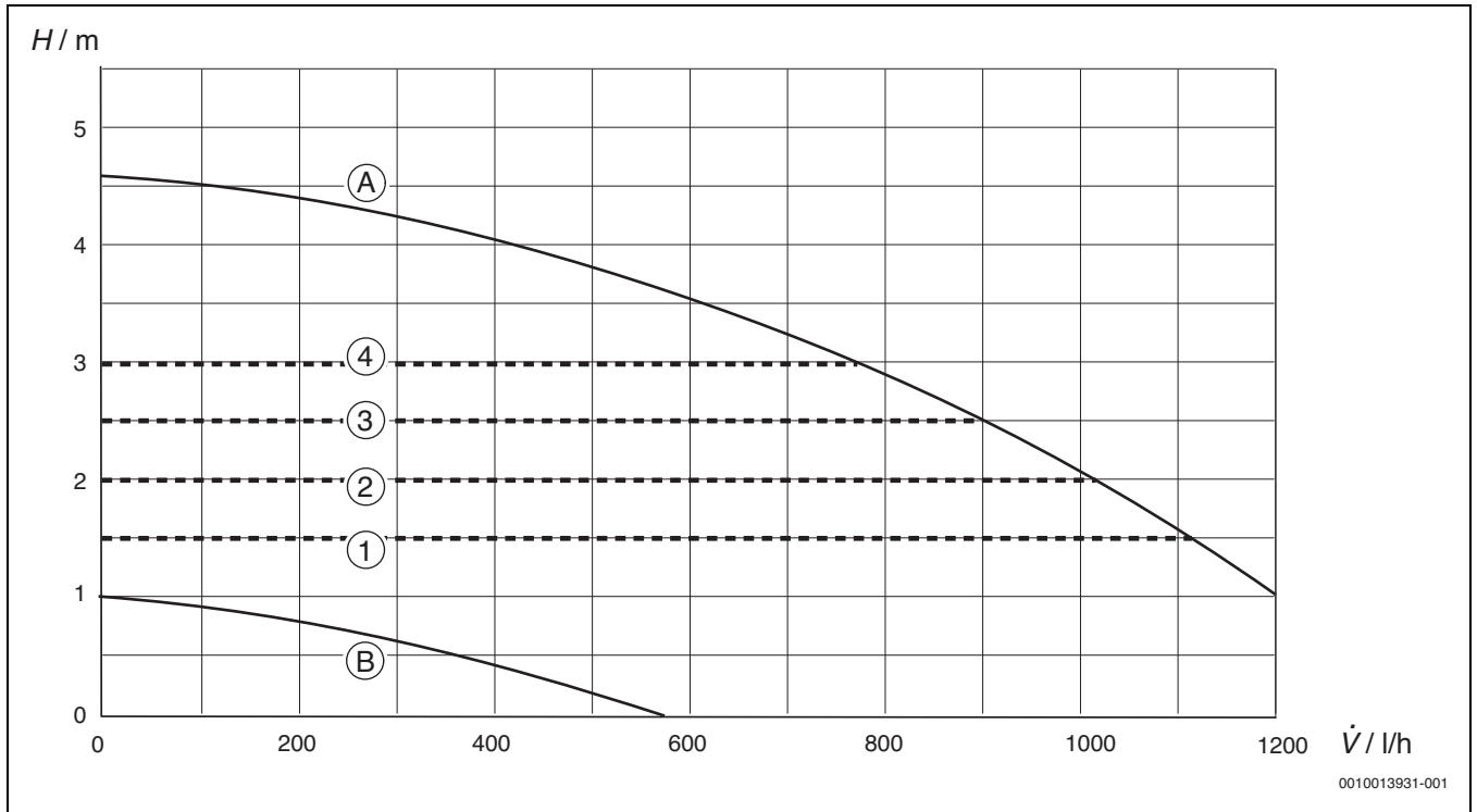
Res. 28 Pompa karakteristik alanları ve pompa eğrileri
