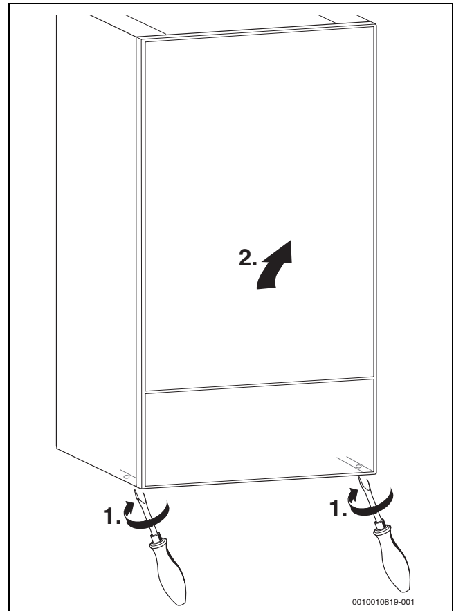
Res. 17 Dış Sacın Çıkartılması
