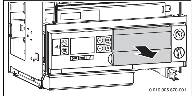
Res. 24 Kapağın çıkarılması ve kumanda panelinin monte edilmesi
