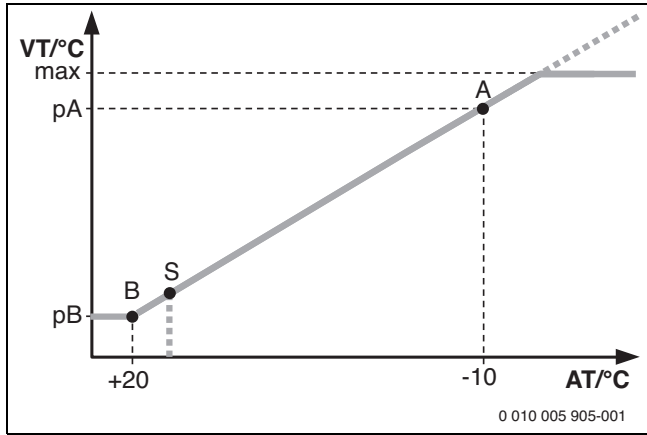
Res. 27 Isıtma eğrisi
