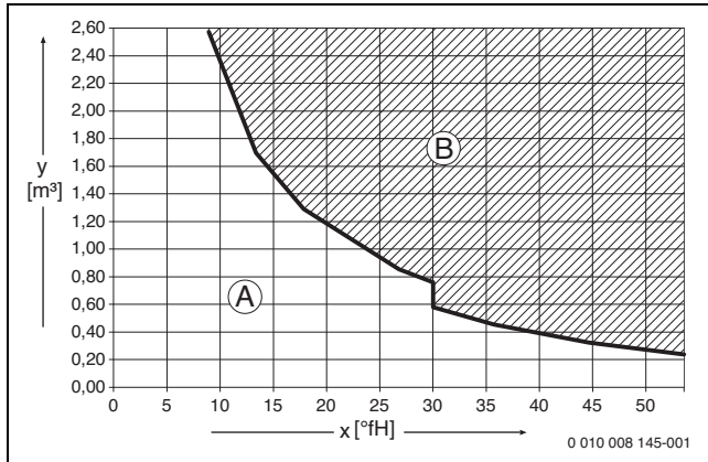
Res. 12 Kapasitesi < 50 kW olan cihazlardaki °fH olarak doldurma ve ekleme suyu ile ilgili gereklilikler
