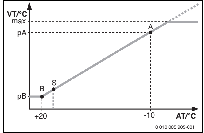
Res. 23 Isıtma eğrisi
