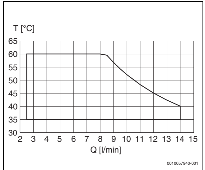
Res. 24 Giriş suyu sıcaklığı 10°C olarak kabul edilmiştir.
