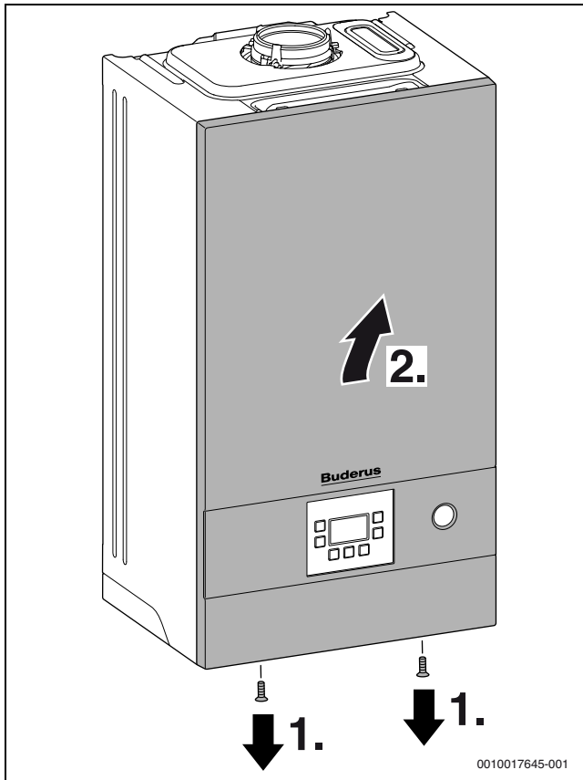
Res. 14 Ön dış sacın çıkarılması
