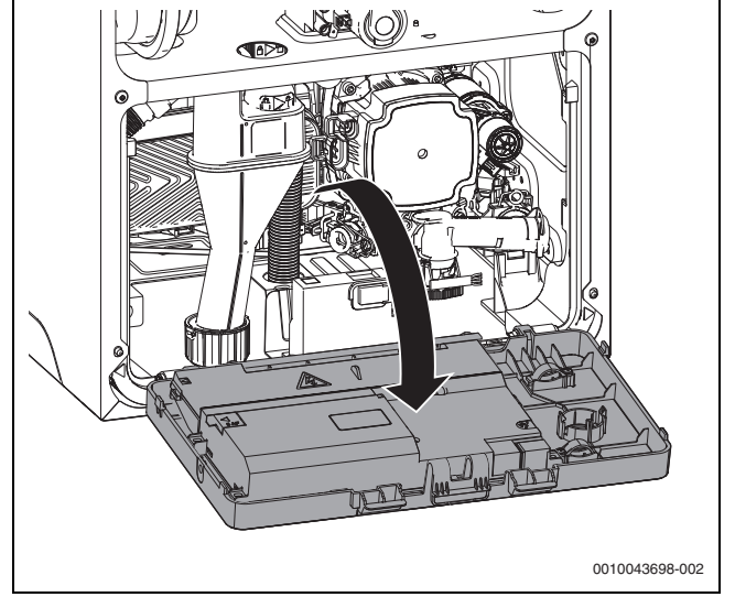
Res. 19 Elektronik sistemin aşağı doğru açılması
