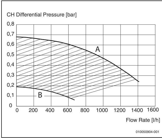
Res. 22 Sirkülasyon pompasının karakteristik eğrisi
