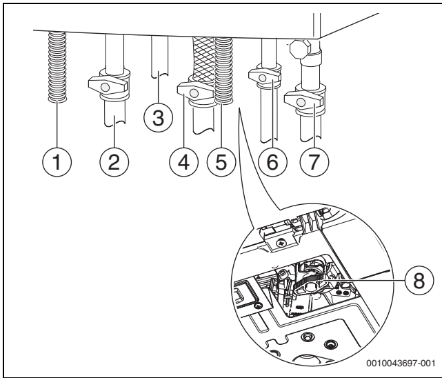
Res. 17 Gaz ve su tarafındaki bağlantılar (aksesuar)
