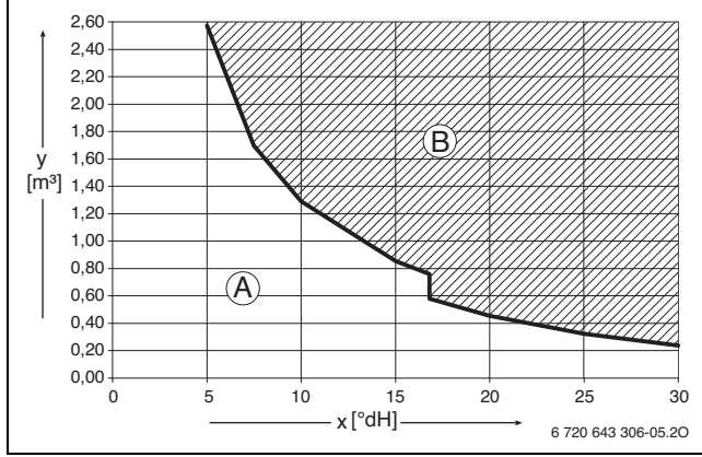
Res. 11 Kapasitesi < 50 kW olan cihazlardaki °dH olarak doldurma ve ekleme suyu ile ilgili gereklilikler
