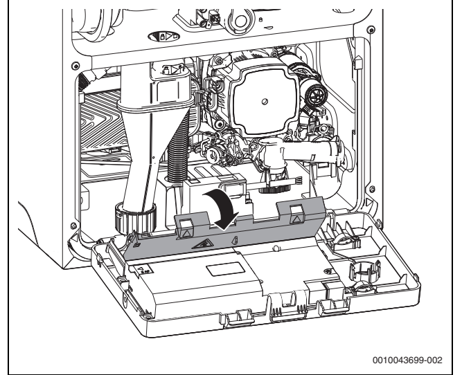
Res. 20 Kapağın açılması
