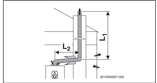
Res. 10 Cihazda oda havasına bağlı hava beslemeli ve kurulum yeri ile havalandırma boşluğu arasında konsantrik bağlantı parçalı, havalandırma boşluğunda B 23p /B 53p uyarınca sabit atık gaz tahliyesi
