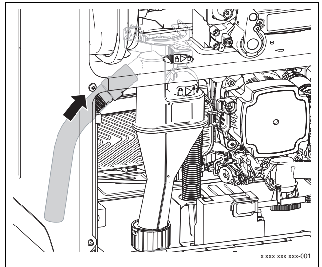
Res. 16 Hortumun yoğuşma suyu sifonuna monte edilmesi
