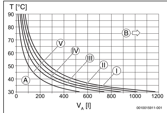
Res. 13 Genleşme tankının karakteristik eğrileri
