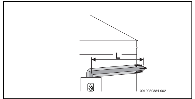
Res. 6 C 13x uyarınca dış duvardan geçen yatay konsantrik hava-atık gaz taşıma sistemi
