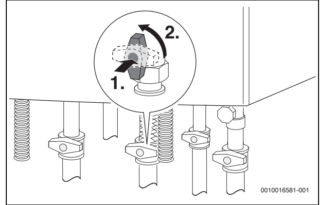
Res. 5 Gaz vanasının açılması
