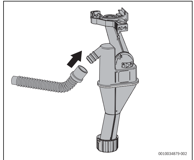
Res. 26 Yoğuşma suyu hortumunun yoğuşma suyu sifonuna monte edilmesi
