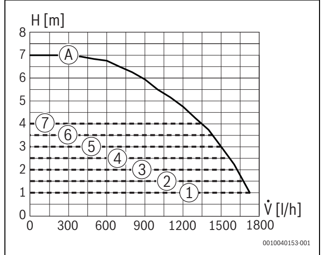
Res. 38 Pompa karakteristik alanları ve pompa karakteristik eğrileri GB172i.2-30 KDW HGB182i.2-35 KW H, GB172i.2-35 KDW HGB182i.2-35 W H, GB172i.2-35 W H, GB172i.2-40 W
