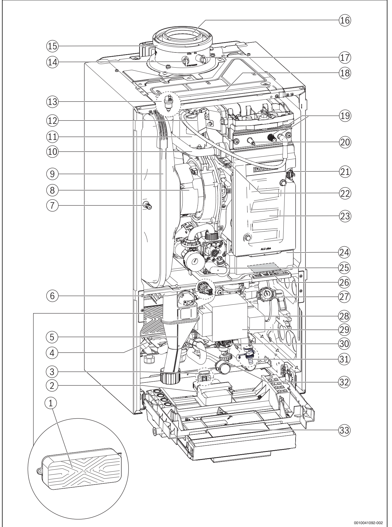
Res. 4 Ürüne genel bakış - Kombi cihazı
