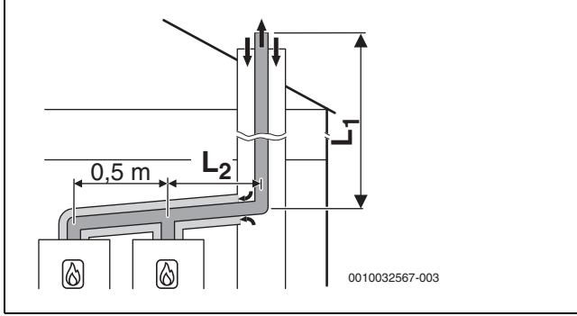
Res. 18 2 cihaz içeren kaskad:
