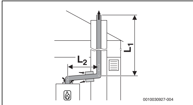
Res. 15 Cihazda oda havasına bağlı hava beslemeli ve kazan dairesi ile havalandırma boşluğu arasında konsantrik bağlantı parçalı, havalandırma boşluğunda B 53p uyarınca sabit atık gaz tahliyesi
