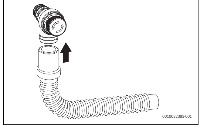
Res. 25 Hortumun emniyet ventiline (ısıtma tesisatı) monte edilmesi
