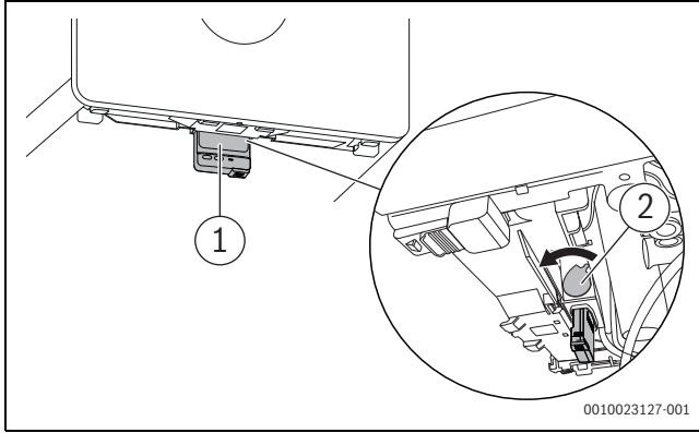
Res. 36 Connect-Key'in sabitlenmesi
