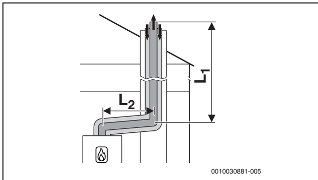
Res. 9 Havalandırma boşluğunda C 33x uyarınca konsantrik hava-atık gaz taşıma sistemi
