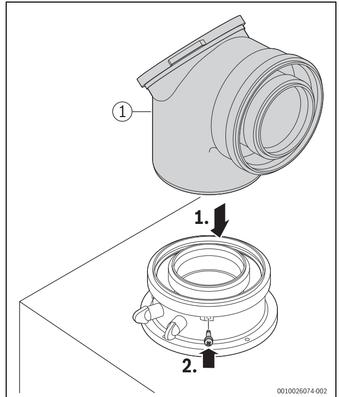
Res. 30 Atık gaz aksesuarının yerleştirilmesi ve vida ile sabitlenmesi
