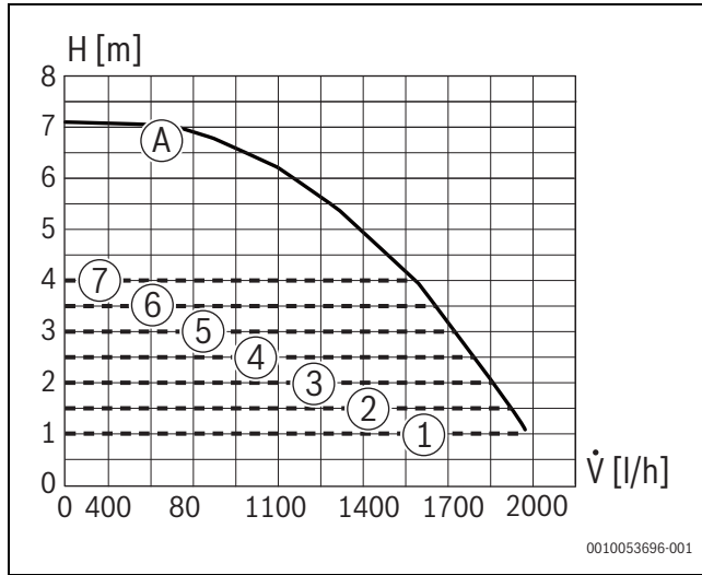
Res. 39 Pompa karakteristik alanları ve pompa karakteristik eğrileri GB172i.2-45 WH
