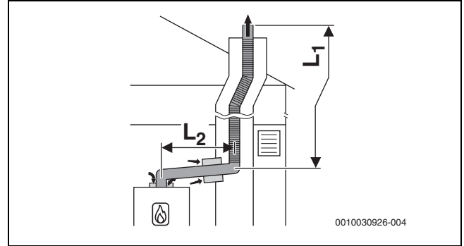
Res. 16 Cihazda oda havasına bağlı hava beslemeli ve kazan dairesi ile havalandırma boşluğu arasında konsantrik bağlantı parçalı, havalandırma boşluğunda B 53p uyarınca esnek atık gaz tahliyesi
