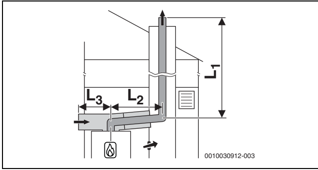
Res. 11 Havalandırma boşluğunda ve ayrı hava beslemeli hava-atık gaz taşıma sisteminde C 53x uyarınca sabit atık gaz tahliyesi ve kazan dairesinde konsantrik atık gaz hattı
