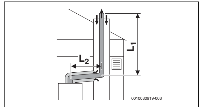
Res. 13 Havalandırma boşluğunda C 93x uyarınca sabit atık gaz tahliyesi ve kurulum yerinde konsantrik hava-atık gaz taşıma sistemi
