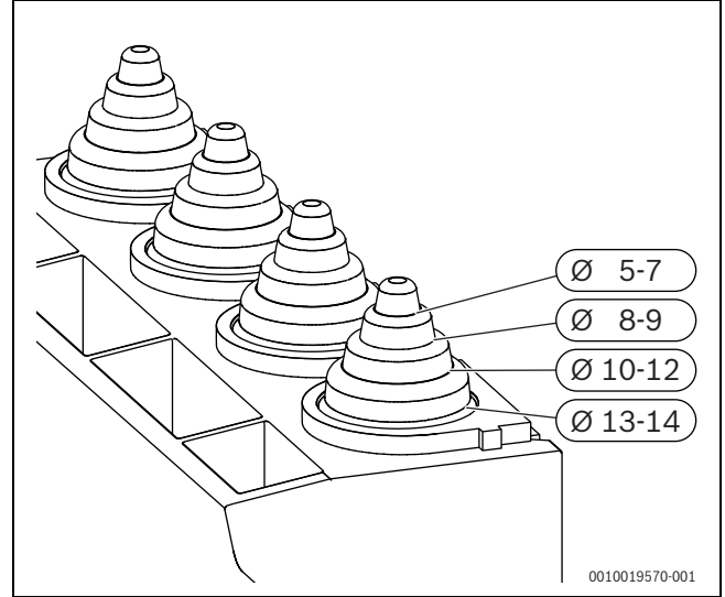
Res. 33 Sabitleme bandının kablo çapına uygun ayarlanması
