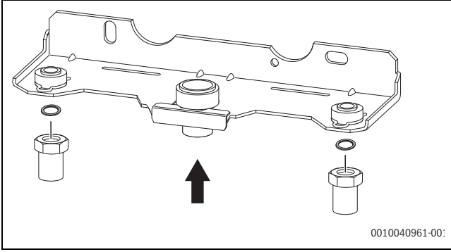
Res. 23 Contalı boruların montaj bağlantı plakasına monte edilmesi
