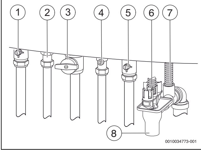
Res. 31 Gaz ve su tarafındaki bağlantılar (aksesuar)
