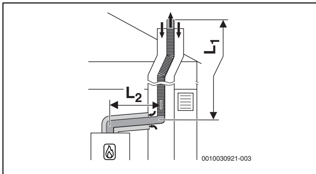
Res. 14 Havalandırma boşluğunda C 93x uyarınca esnek atık gaz tahliyesi ve kurulum yerinde konsantrik hava-atık gaz taşıma sistemi
