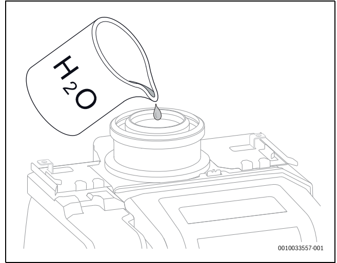
Res. 29 Yoğuşma suyu sifonuna su doldurulması
