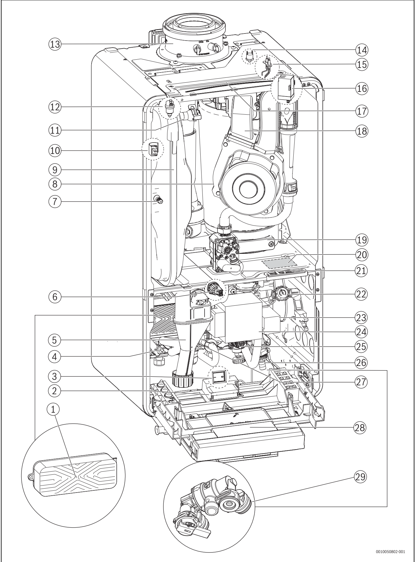
Res. 4 Ürüne genel bakış
