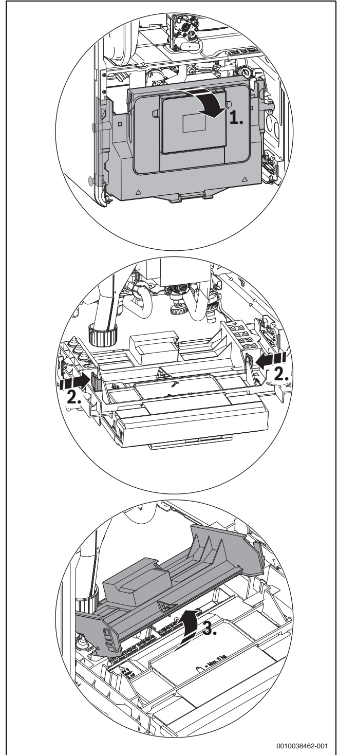
Res. 25 Kapağın açılması
