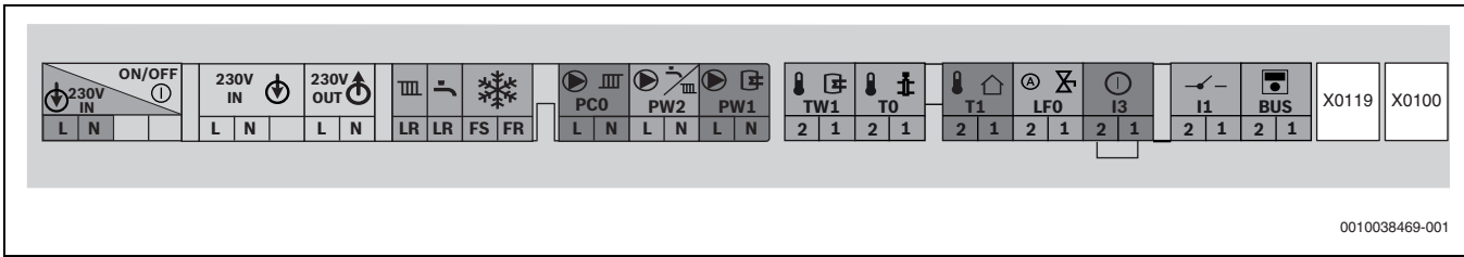
Res. 27 Harici aksesuar için terminal bloğu
