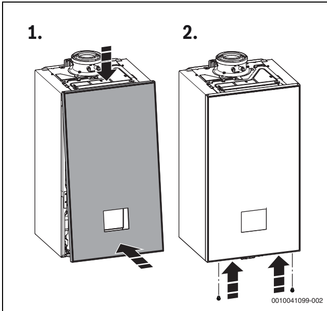
Res. 28 Dış panelin monte edilmesi
