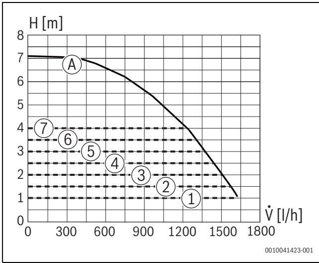
Res. 29 Pompa karakteristik alanları ve pompa karakteristik eğrileri
