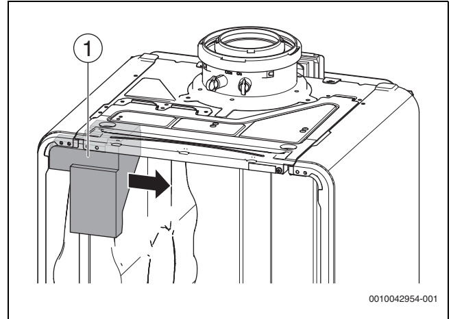
Res. 19 Destek süngerinin çıkarılması
