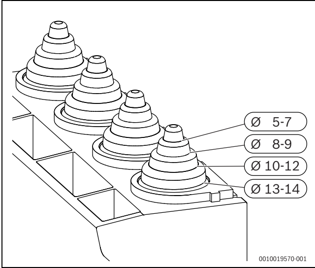
Res. 26 Sabitleme bandının kablo çapına uygun ayarlanması
