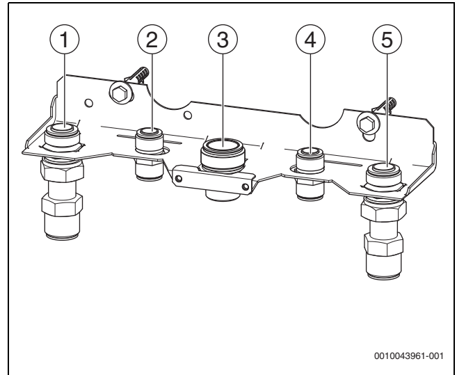
Res. 24 Gaz ve su tarafındaki bağlantılar
