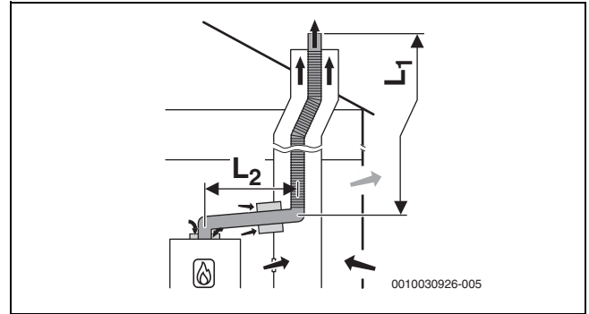
Res. 13 Cihazda oda havasına bağlı hava beslemeli ve kurulum yerinde tek cidarlı atık gaz hattı, havalandırma boşluğunda B 53p uyarınca esnek atık gaz tahliyesi; havalandırma boşluğunda arka havalandırma açıklığı
