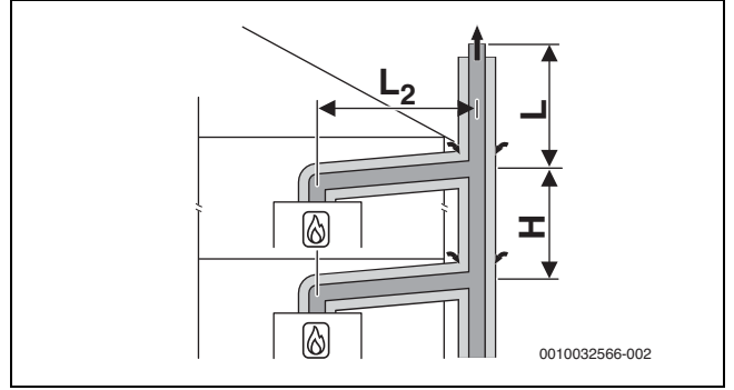
Res. 14 Dış duvarda ve kazan dairesinde konsantrik hava-atık gaz taşıma sistemi C (13)3x uyarınca çoklu bağlantı
