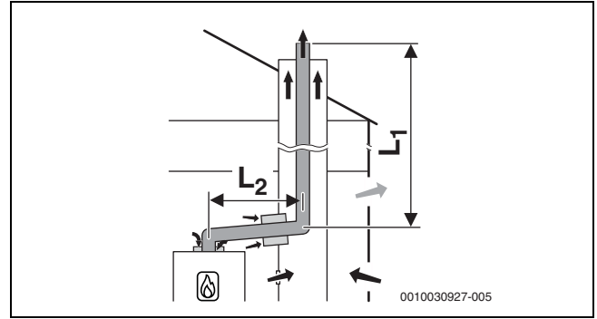
Res. 12 Cihazda oda havasına bağlı hava beslemeli ve kurulum yerinde tek cidarlı atık gaz hattı, havalandırma boşluğunda B 53p uyarınca sabit atık gaz tahliyesi; havalandırma boşluğunda arka havalandırma açıklığı
