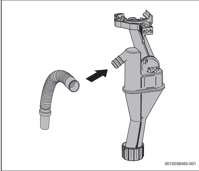
Res. 21 Yoğuşma suyu hortumunun bağlantı parçasına takılması
