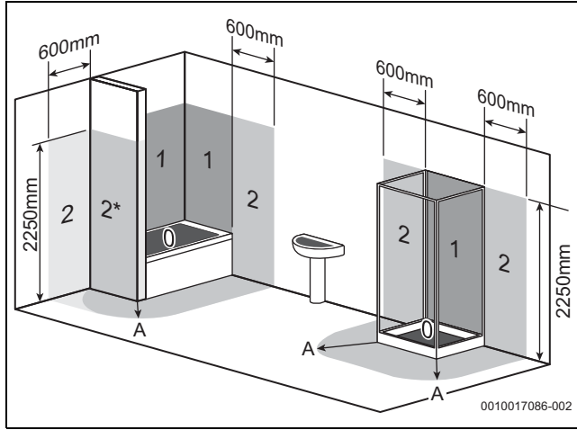
Res. 15 Koruma alanları (örnek gösterim)
