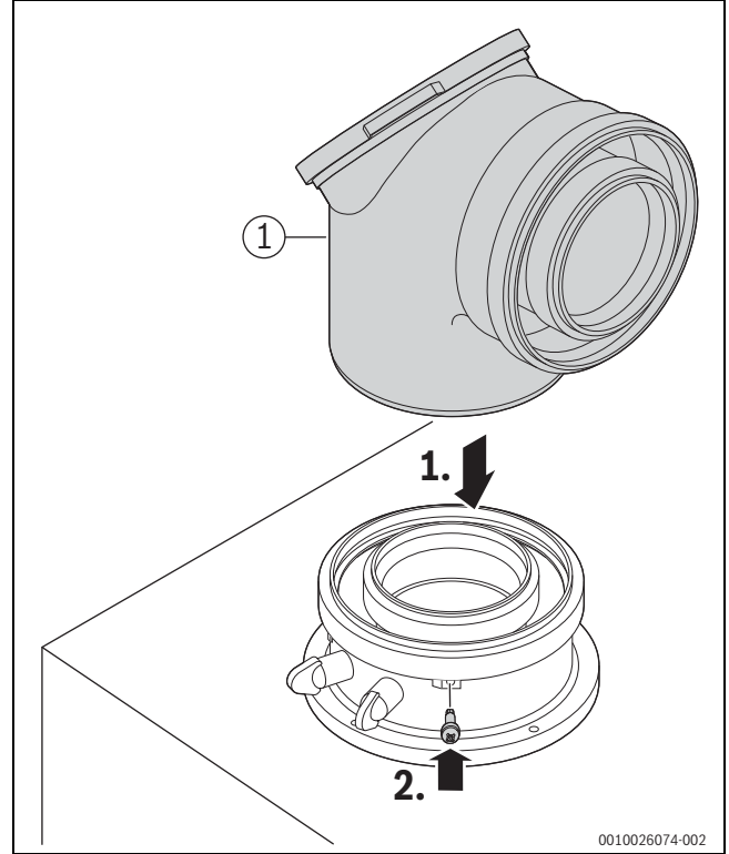
Res. 23 Atık gaz aksesuarının yerleştirilmesi ve vida ile sabitlenmesi
