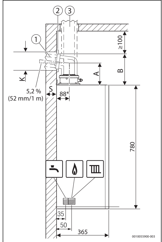
Res. 2 Yandan görünüm (mm)
