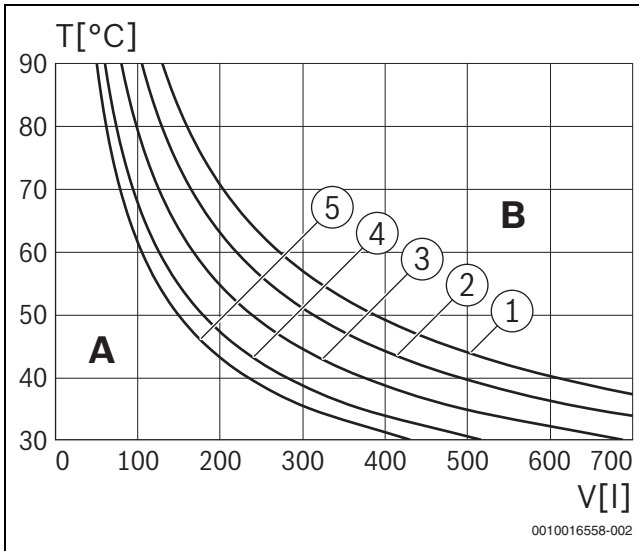
Res. 18 Genleşme tankının karakteristik eğrileri
