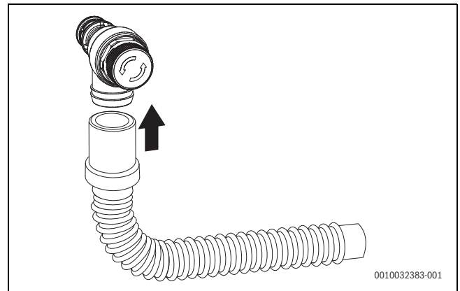
Res. 20 Hortumun emniyet ventiline (ısıtma tesisatı) monte edilmesi
