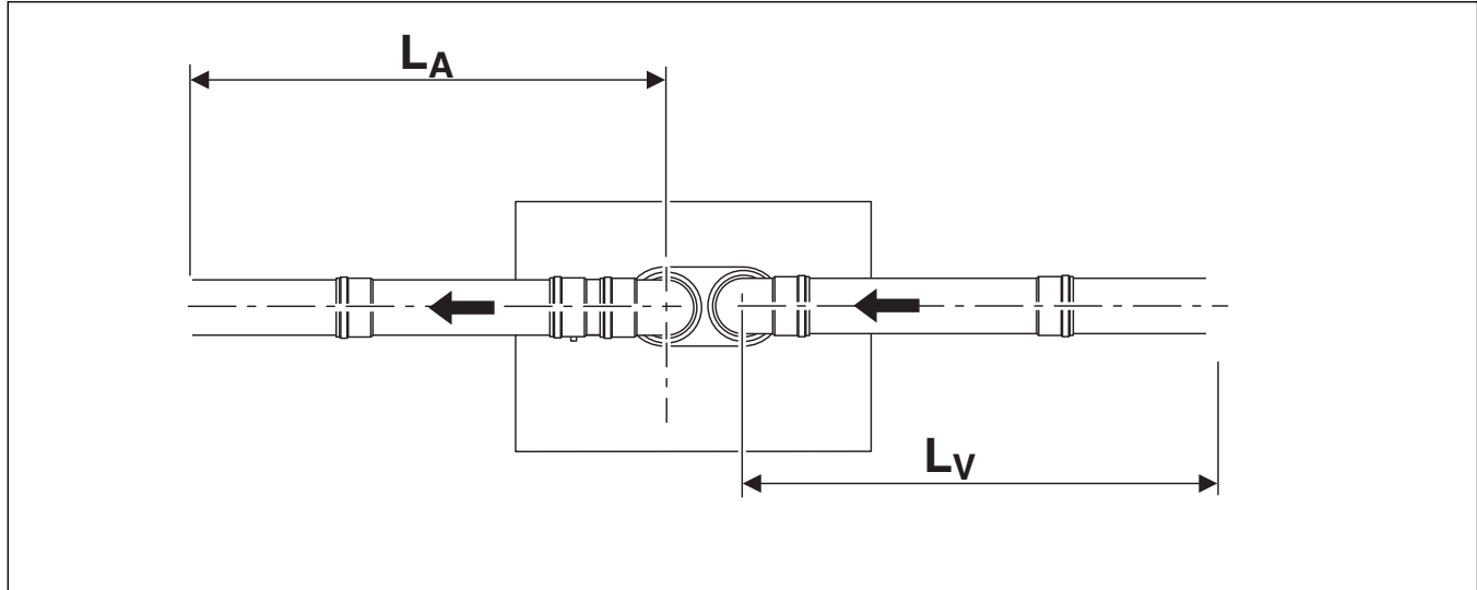
Res. 14 C 52 / C 82 Yatay Tip Bağlantı Örneği
