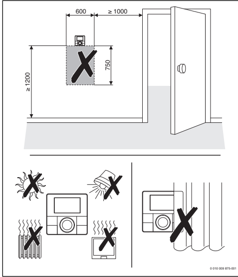
Res. 6 Referans odasındaki montaj yeri
