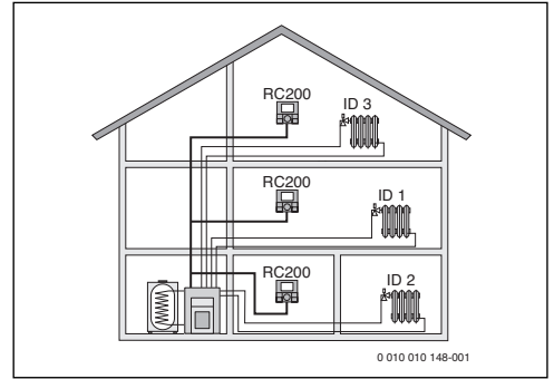
Res. 3 Kumanda cihazı olarak her birinde bir RC200 mevcut üç ısıtma devreli ısıtma tesisatı için (apartman) örnek
