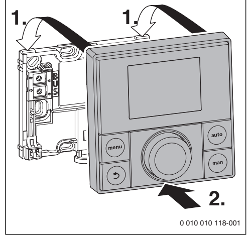
Res. 9 Kumanda panelinin asılması
