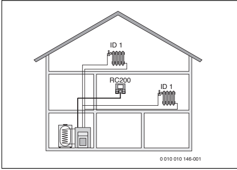
Res. 1 Tek HK 1 ısıtma devreli ve kontrol ünitesi olarak RC200 kumanda paneli donanımlı bir ısıtma tesisatı örneği (müstakil ev)
