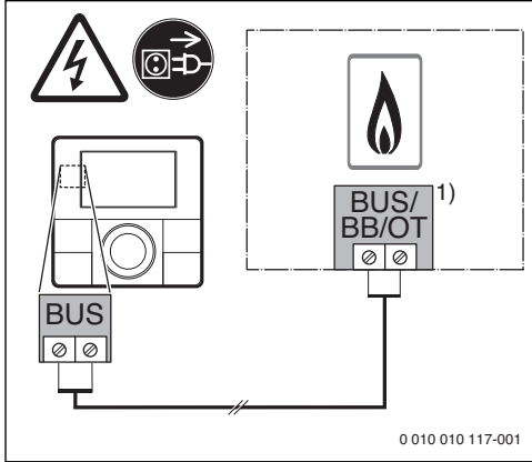
Res. 8 Kumanda panelinin bir ısıtma cihazına bağlanması
