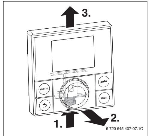
Res. 10 Kumanda panelinin yerinden çıkartılması
