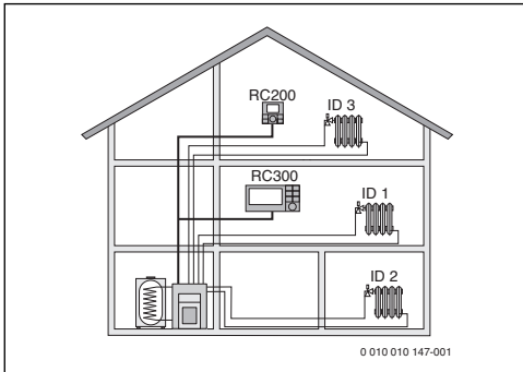
Res. 2 Üç ısıtma devreli ve uzaktan kumanda olarak kullanılan RC200 donanımlı bir ısıtma tesisatı örneği (kiralık odalı veya atölyeli müstakil ev)
