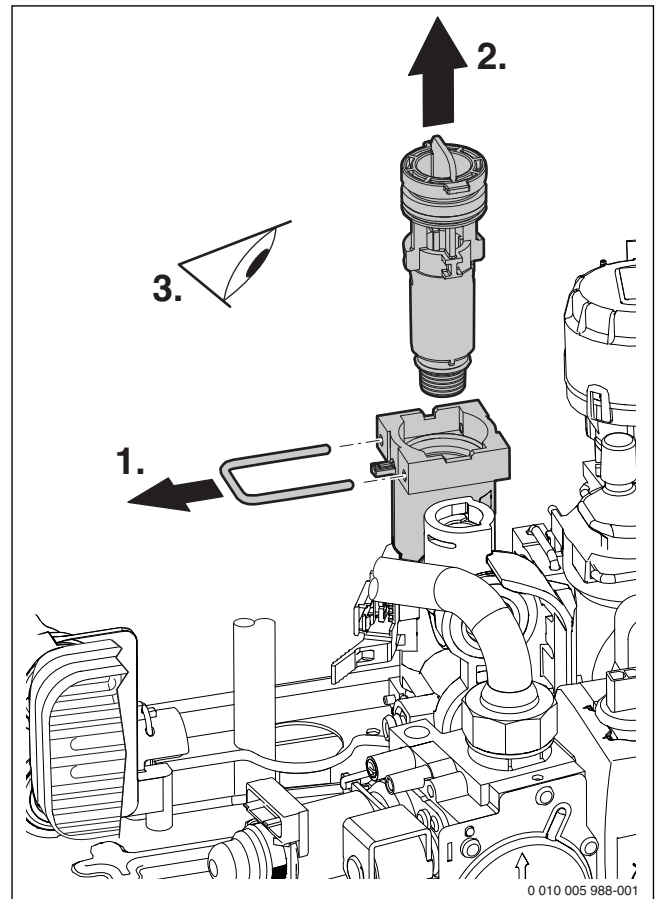
Res. 34 Soğuk su borusundaki filtrenin kontrol edilmesi
