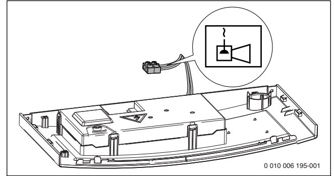
Res. 23 Alarm kontağının bağlanması
