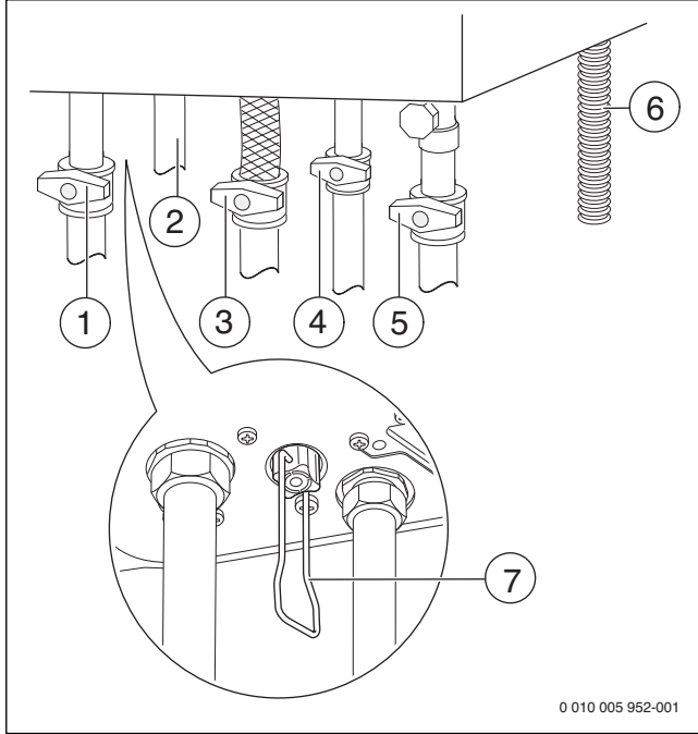
Res. 19 Gaz ve su tarafı bağlantıları (aksesuar)
