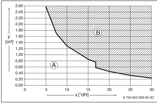
Res. 11 Kapasitesi < 50 kW olan cihazlardaki doldurma ve ekleme suyu ile ilgili gereklilikler
