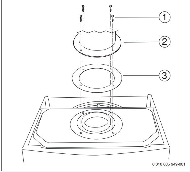
Res. 16 Atık gaz aksesuarının tespit edilmesi
