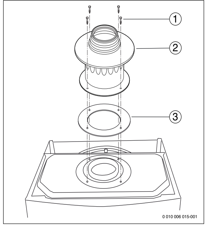
Res. 18 B 22 dikey atık gaz tahliyesinde ve cihaz kapasitesi = 35 kW olduğunda: Atık gaz adaptörü ve kısma plakası monte edilmelidir
