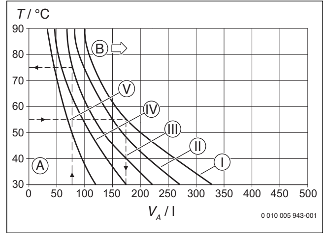
Res. 12 Genleşme tankının karakteristik eğrileri
