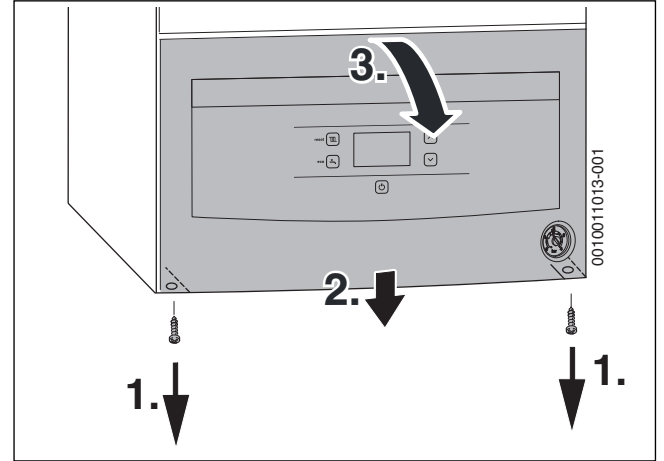
Res. 15 Kumanda cihazının aşağı doğru açılması
