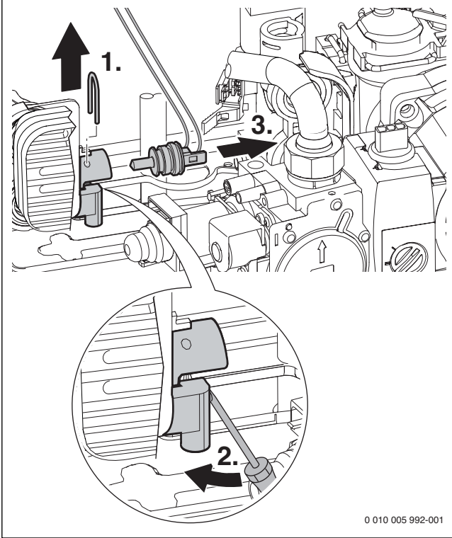
Res. 38 Kullanım suyu sıcaklık sensörünün sökülmesi
