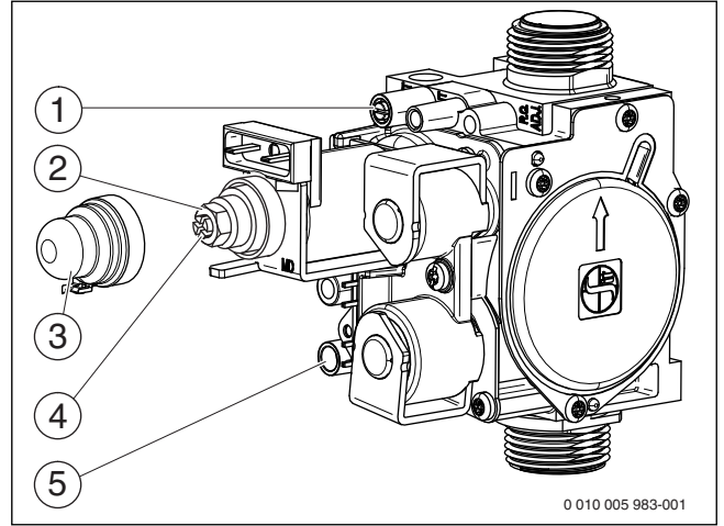
Res. 30 Gaz armatürü
