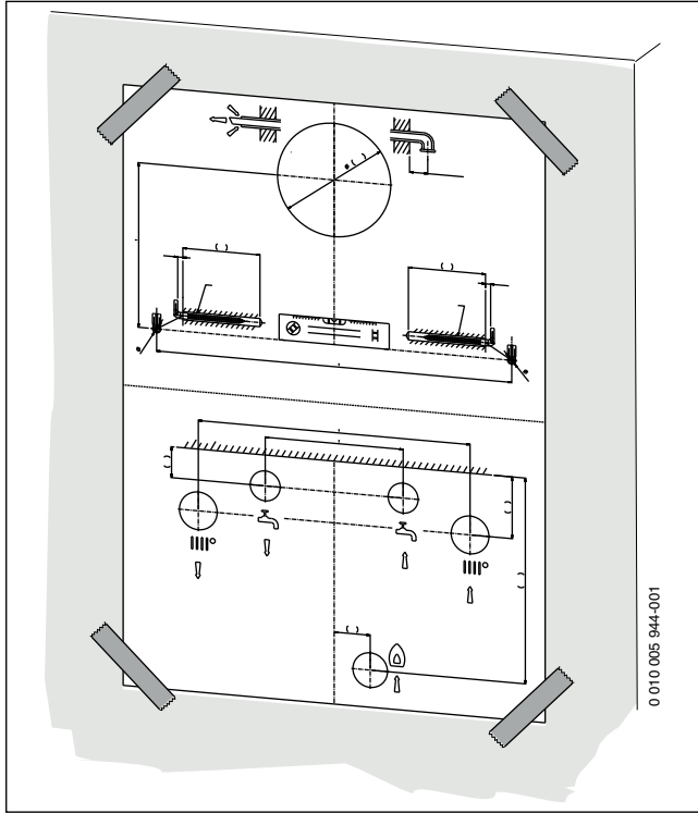
Res. 13 Montaj şablonu
