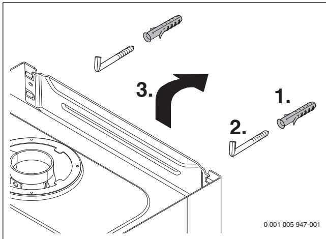
Res. 14 Cihazın kancalı vidalara asılması
