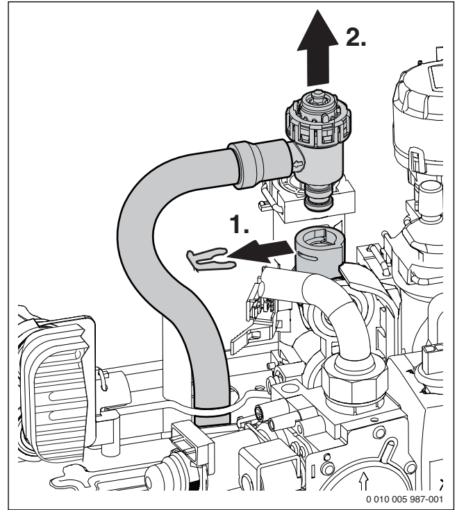
Res. 33 Emniyet ventilinin (ısıtma devresi) çıkarılması
