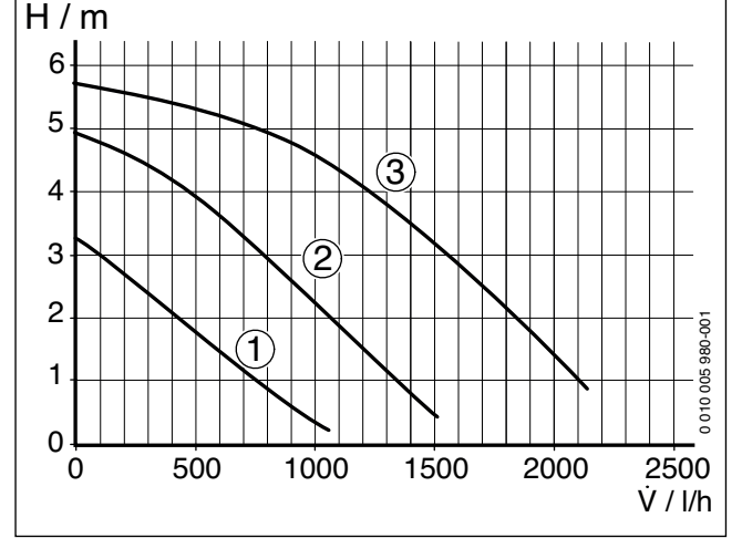
Res. 27 Sirkülasyon pompası karakteristik eğrisi (cihaz kapasitesi < 35 kW)
