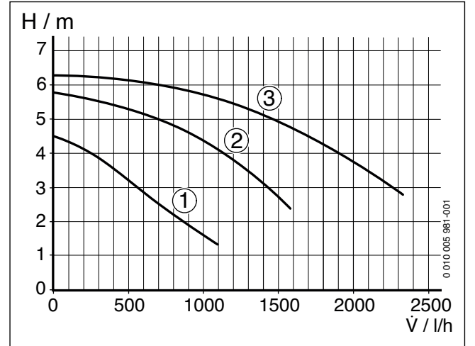
Res. 28 Sirkülasyon pompası karakteristik eğrisi (cihaz kapasitesi = 35 kW)
