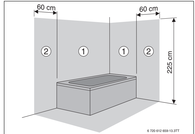
Res. 20 Koruma alanları
