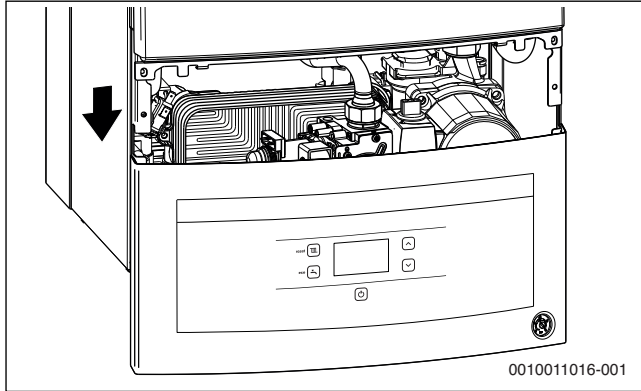
Res. 29 Gaz armatürünü ve kumanda cihazını aynı anda kullanabilmek için çerçeveye asılmış kumanda cihazı
