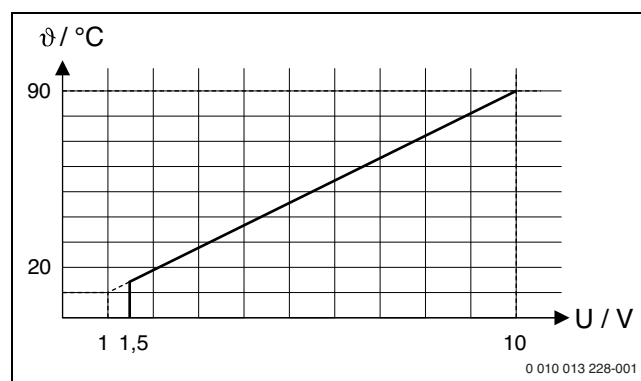
Fig. 9 Lineær sammenhæng mellem 0-10 V signalet (U i volt) og den krævede fremløbstemperatur θ (i °C baseret på området minimal fremløbstemperatur til maksimal fremløbstemperatur [grundindstilling 20 °C til 90 °C])
