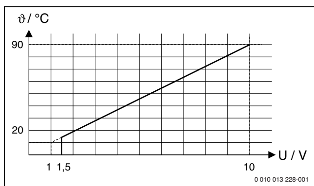
Rys. 37 Liniowa zależność między sygnałem 0–10 V ( U w voltach) a żadaną temperaturą zasilania \theta (w °C w stosunku do zakresu od minimalnej temperatury zasilania do maksymalnej temperatury zasilania [ustawienie podstawowe 20 °C do 90 °C])
