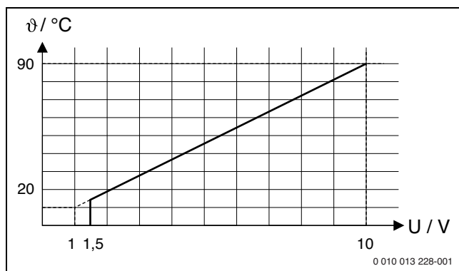
Σχ. 16 Γραμμική συσχέτιση μεταξύ του σήματος 0-10V (U σε Volt) και της ζητούμενης θερμοκρασίας προσαγωγής θ (σε °C σε σχέση με την περιοχή ελάχιστης θερμοκρασίας προσαγωγής μέχρι τη μέγιστη θερμοκρασία παροχής [εργοστασιακή ρύθμιση 20 °C έως 90 °C])
