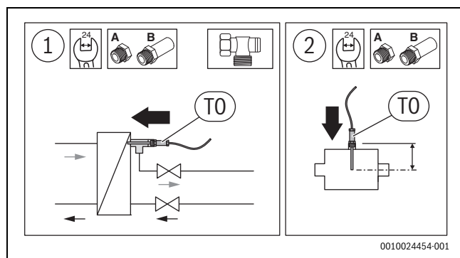
Fig. 10 Optimal følermontering
