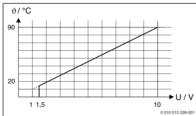
Obr. 44 Lineárna závislosť medzi 0-10V signálom ( U vo Voltch) a požadovanou teplotou výstupu \theta (v °C vo vzťahu k rozsahu minimálnej teploty výstupu až maximálnej teploty výstupu [základné nastavenie 20 °C až 90 °C])
