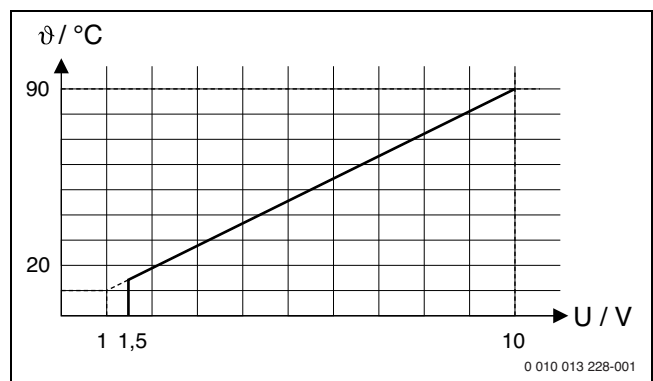
Kuva 23 Lineaarinen yhteys 0-10V-signaalin (U / voltti) ja pyydetyn esilämpötilan θ välillä (°C laitteiston minimin tulolämpötilan alueen suhteen maksimiin menolämpötilaan asti [perusasetus 20 °C ... 90 °C])
