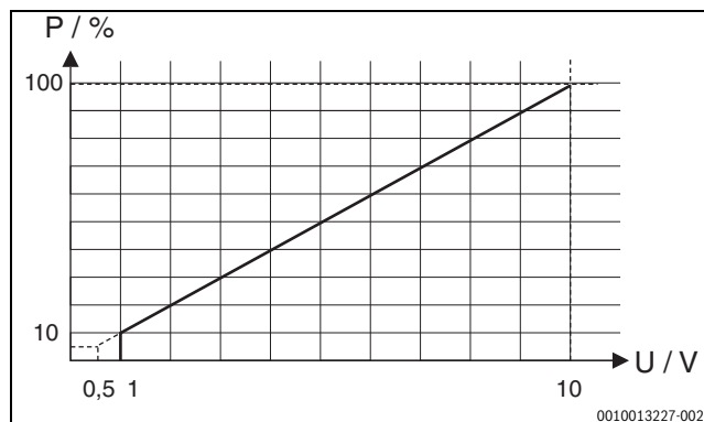
Obr. 43 Lineárna závislosť medzi 0-10 V signálom ( U vo Voltch) a požadovaným výkonom P (v percentách vo vzťahu k maximálnemu výkonu zariadenia)
