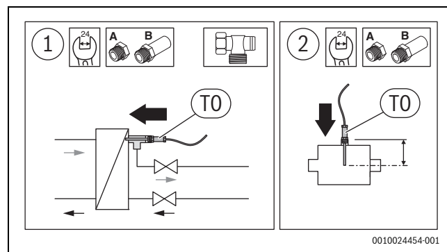
Rys. 38 Optymalny montaż czujnika
