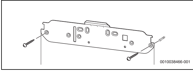
Res. 19 Askı aparatının monte edilmesi
