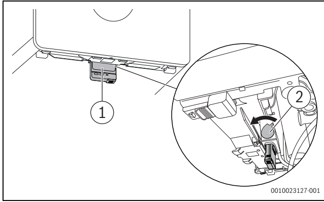
Res. 33 Connect-Key'in sabitlenmesi
