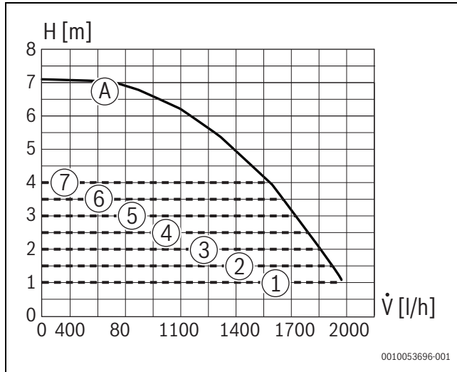
Res. 36 Pompa karakteristik alanları ve pompa karakteristik eğrileri GB172i.2-45 WH
