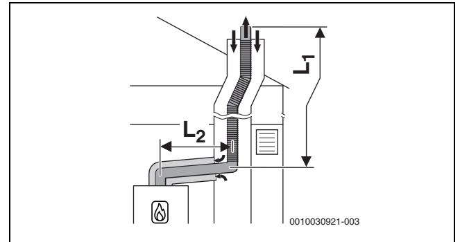
Res. 12 Havalandırma boşluğunda C 93x uyarınca esnek atık gaz tahliyesi ve kurulum yerinde konsantrik hava-atık gaz taşıma sistemi
