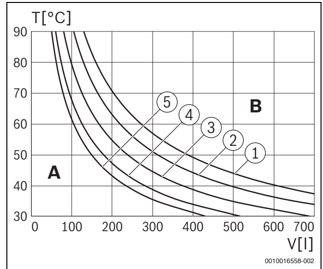
Res. 18 Genleşme tankının karakteristik eğrileri
