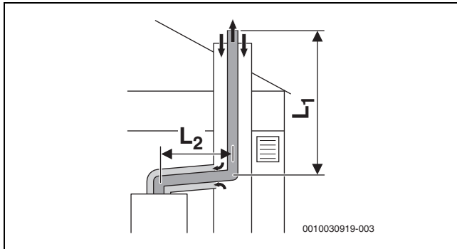
Res. 11 Havalandırma boşluğunda C 93x uyarınca sabit atık gaz tahliyesi ve kurulum yerinde konsantrik hava-atık gaz taşıma sistemi
