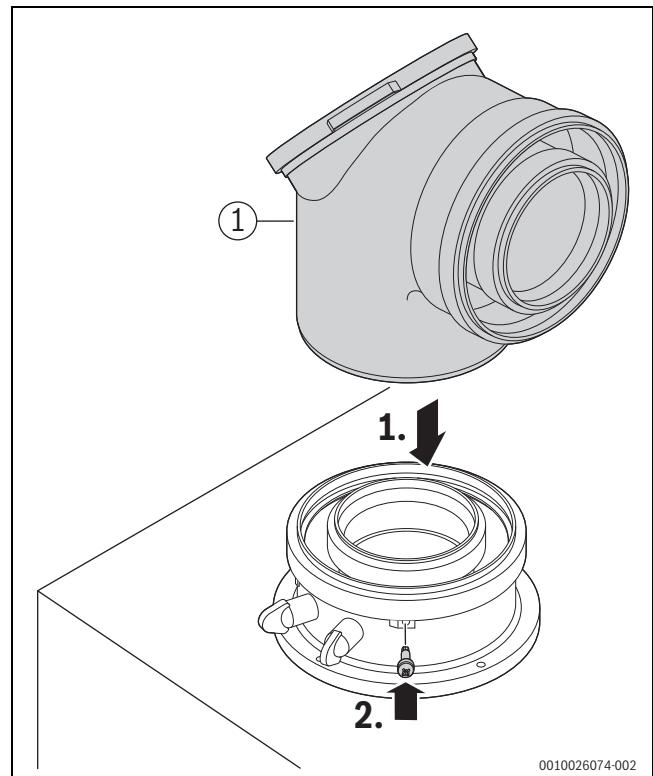
Res. 27 Atık gaz aksesuarının yerleştirilmesi ve vida ile sabitlenmesi
