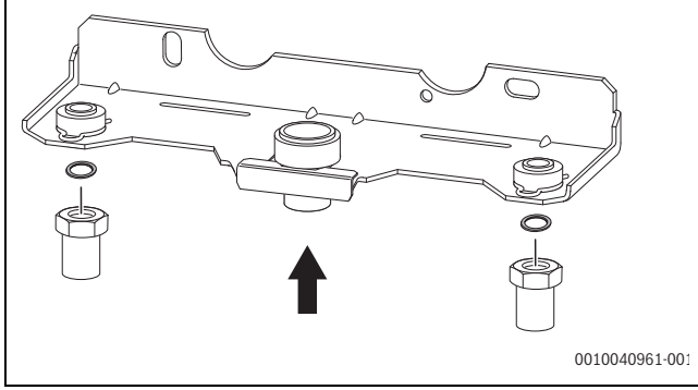
Res. 20 Contalı boruların montaj bağlantı plakasına monte edilmesi
