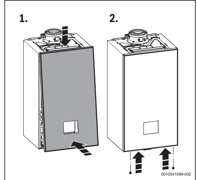
Res. 34 Dış panelin monte edilmesi
