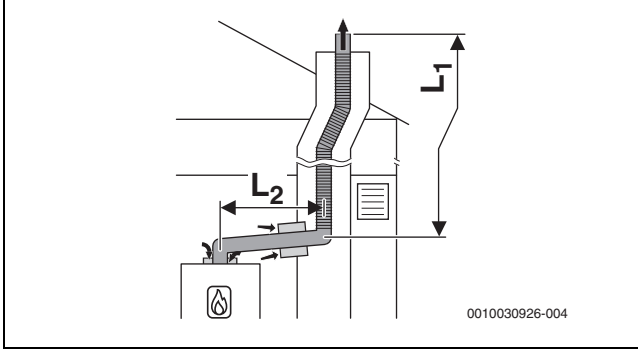
Res. 14 Cihazda oda havasına bağlı hava beslemeli ve kazan dairesi ile havalandırma boşluğu arasında konsantrik bağlantı parçalı, havalandırma boşluğunda B 53p uyarınca esnek atık gaz tahliyesi
