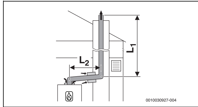
Res. 13 Cihazda oda havasına bağlı hava beslemeli ve kazan dairesi ile havalandırma boşluğu arasında konsantrik bağlantı parçalı, havalandırma boşluğunda B 53p uyarınca sabit atık gaz tahliyesi
