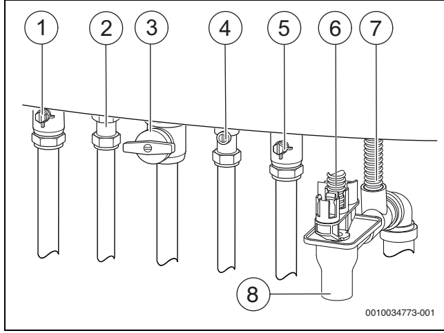
Res. 28 Gaz ve su tarafındaki bağlantılar (aksesuar)
