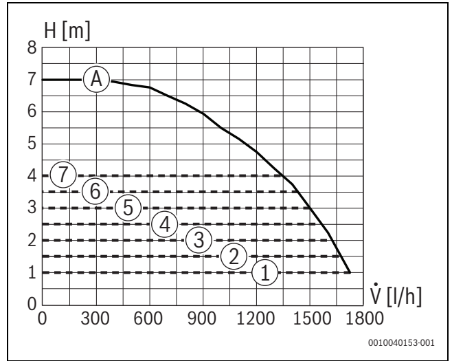
Res. 35 Pompa karakteristik alanları ve pompa karakteristik eğrileri GB172i.2-30 KDW HGB182i.2-35 KW H, GB172i.2-35 KDW HGB182i.2-35 W H, GB172i.2-35 W H, GB172i.2-40 W
