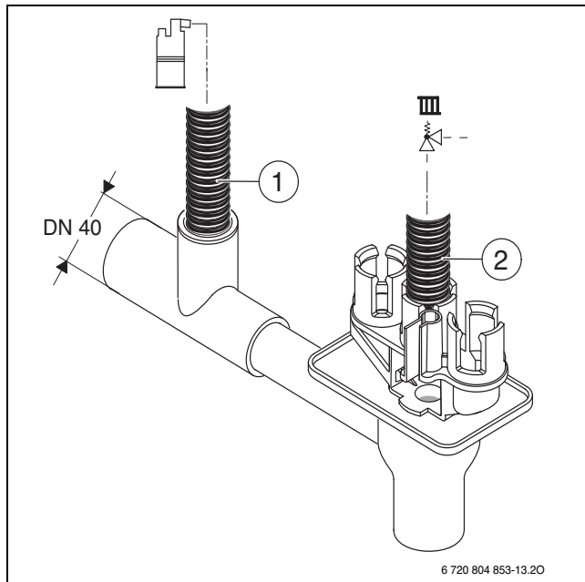
Res. 24 Kondens suyu hortumunun ve emniyet ventiliinden gelen hortumun sifona monte edilmesi
