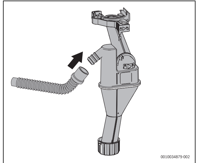
Res. 23 Yoğuşma suyu hortumunun yoğuşma suyu sifonuna monte edilmesi
