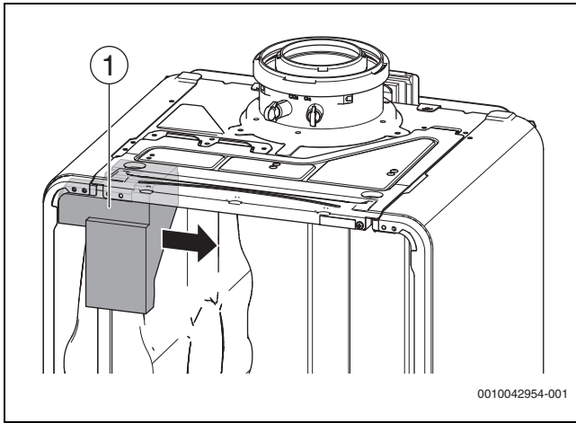
Res. 21 Destek süngerinin çıkarılması
