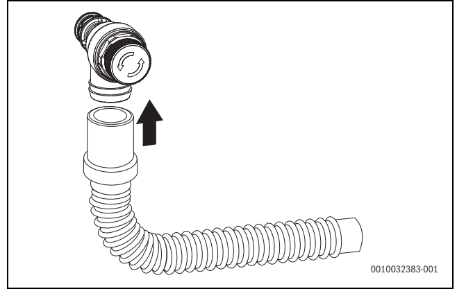
Res. 22 Hortumun emniyet ventiline (ısıtma tesistatı) monte edilmesi
