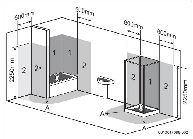
Res. 15 Koruma alanları (örnek gösterim)
